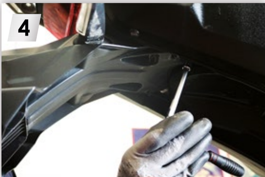
4 4 x Halteschrauben SW8 entfernen. Remove 4 x SW8 retaining screws.
