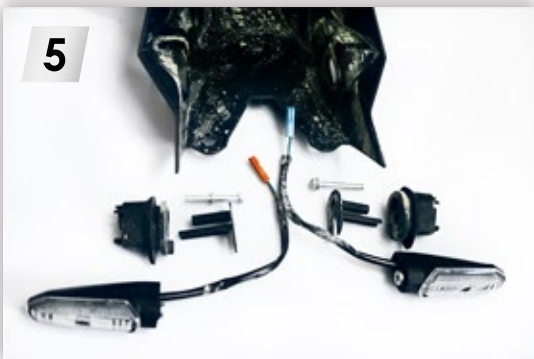
5 Die originalen Blinker demontieren. Remove the original indicators.
